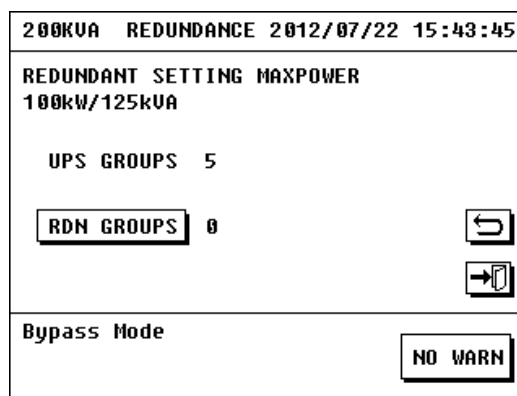
Рис. 3.43 Настройка избыточности
