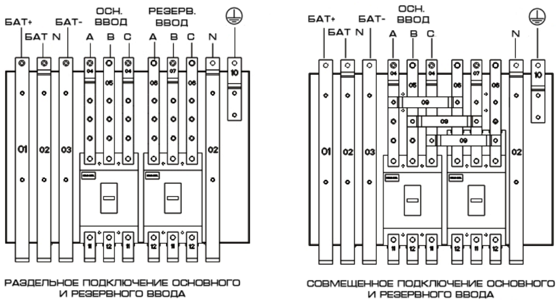
Рис. 2.15 Входные и выходные подключения кабинета 160кВА
