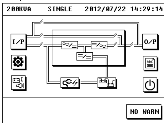
Рис. 3.7 Главное меню.
