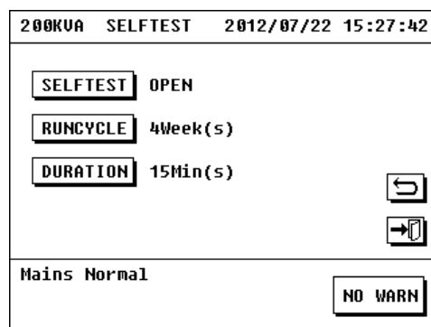
Рис. 3.42 Настройка самодиагностики
