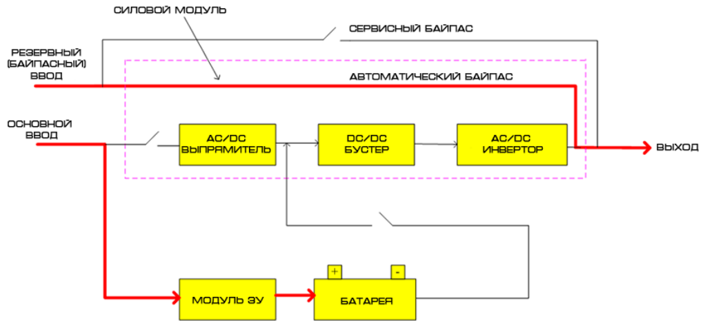
Рис. 1.5 Диаграмма работы одного модуля в байпасном режиме
